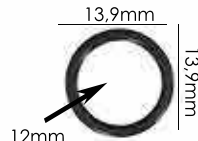
Ref.: APA 002/A 12mm Espessura: 1,3mm Materiais: POM, PP e PC Embalagem: 1000 unidades
