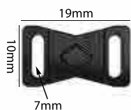
Ref.: APF 000 7mm Espessura: 2,2mm Materiais: POM, PC e HS Embalagem: 1000 unidades
