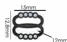
Ref.: APR 005 12mm Espessura: 1,8mm Materiais: POM e PC Acabamentos: Cristal ou Oktant Swarovski Embalagem: 100 unidades
