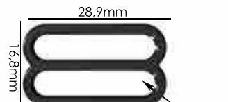
Ref.: APR 017 24,5mm Espessura: 2,1mm Materiais: POM e PC Embalagem: 1000 unidades
