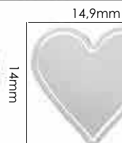
Ref.: AML CORAÇÃO Passante interno: 12,8mm Material: zamac Espessura: 4,5mm
