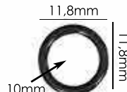
Ref.: APA 001/A 10mm Espessura: 1,3mm Materiais: POM, PP, PC e HC Embalagem: 1000 unidades
