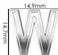
Ref.: AML W Passante interno: 12mm Material: zamac Espessura: 4,5mm
