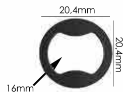
Ref.: APA 011 PARALELA 16mm Espessura: 1,5mm Materiais: POM, PP e PC Embalagem: 1000 unidades
