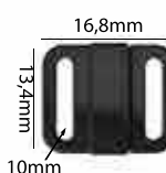
Ref.: APF 006 10mm Espessura: 4,5mm Materiais: POM, PC e HS Embalagem: 1000 unidades
