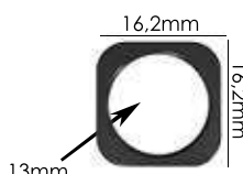
Ref.: APA 007 13mm Espessura: 1,5mm Materiais: POM, PC e HS Embalagem: 1000 unidades
