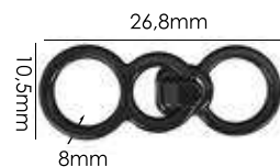
Ref.: APF 004 8mm Espessura: 4,8mm Materiais: POM, PC e HS Embalagem: 1000 unidades
