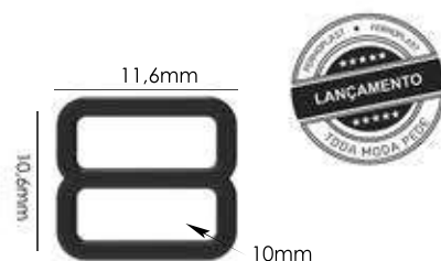
Ref.: APR 024 10mm Espessura: 1.3mm Materiais: POM Embalagem: 1000 unidades
