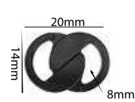
Ref.: APF 015 8mm Espessura: 2,4mm Materiais: POM, PC e HS Embalagem: 1000 unidades
