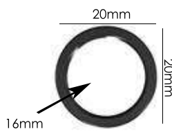
Ref.: APA 008 16mm Espessura: 1,6mm Materiais: POM, PC e HS Embalagem: 1000 unidades
