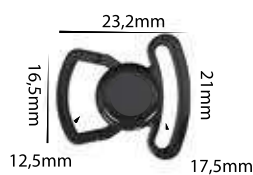
Ref.: APF 034 12,5X17,5mm Espessura: 4,2mm Materiais: POM Embalagem: 1000 unidades
