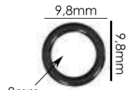
Ref.: APA 000/B 8mm Espessura: 1,3mm Materiais: POM, PP e PC Embalagem: 1000 unidades
