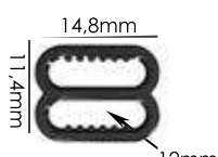
Ref.: APR 015 12mm Espessura: 1,6mm Materiais: POM e PC Embalagem: 1000 unidades
