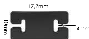
Ref.: APR 021 4mm Espessura: 1,4mm Materiais: POM e PC Embalagem: 1000 unidades
