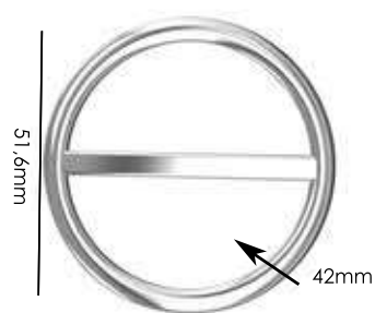
Ref.: AMA 42mm C/ TRAVA
