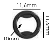
Ref.: APA 001 10mm Espessura: 1,3mm Materiais: POM, PP e PC Embalagem: 1000 unidades
