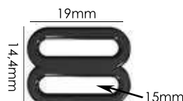
Ref.: APR 004 15mm Espessura: 1,9mm Materiais: POM, PP, PC e HS Embalagem: 1000 unidades
