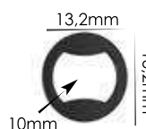
Ref.: APA 009 PARALELA 10mm Espessura: 1,2mm Materiais: POM Embalagem: 1000 unidades
