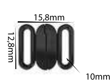
Ref.: APF 019 10mm Espessura: 2,5mm Materiais: POM, PC e HS Embalagem: 1000 unidades
