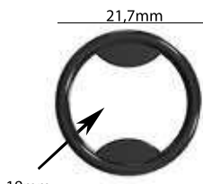
Ref.: APA 005 18mm Espessura: 1,9mm Materiais: POM e PC Embalagem: 1000 unidades
