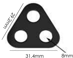
Ref.: APT 3F 8mm Espessura: 2,3mm Materiais: POM, PC e HS Embalagem: 200 unidades
