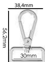
Ref.: AMMQ 004 30mm Material: zamac Banho: Ouro 24K, Ouro Rosé, Níquel Ouro Velho, Cobre, Latão, Onix, Silver, Prata Velho, Dourado e Light Gold Matte. Espessura: 5,6mm. I Embalagem: 100
