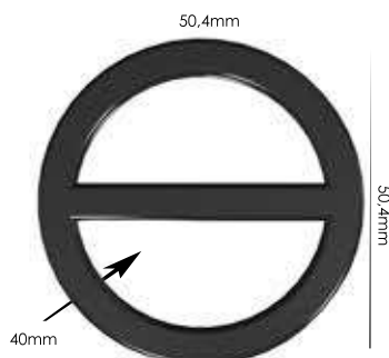
Ref.: APA PARALELA C/ TRAV 40MM Espessura: 2,4mm Materiais: POM, PC e HS Embalagem: 200 unidades
