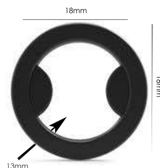
Ref.: APA 021 13mm Espessura: 1,4mm Materiais: POM e PP Embalagem: 1000 unidades
