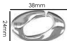
Ref.: AMD 002 24x38mm Material: zamac Banho: Ouro 24K, Ouro Rosé, Níquel Ouro Velho, Cobre, Latão, Onix, Silver, Prata Velho, Dourado e Light Gold Matte. Espessura: 2,2mm. I Embalagem: 100
