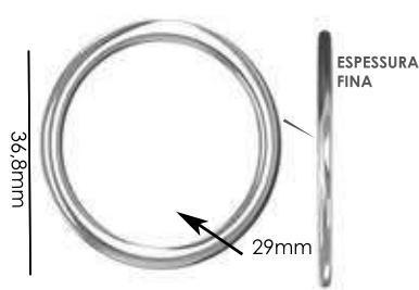
Ref.: AMA 27mm trab (Sob Consulta) Ref.: AMA 29mm
