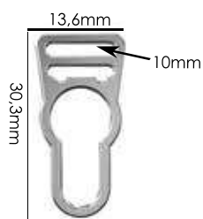
Ref.: AMESP 001 10mm Material: zamac Banho: Ouro 24K, Ouro Rosé, Níquel Ouro Velho, Cobre, Latão, Onix, Silver, Prata Velho, Dourado e Light Gold Matte. Espessura: 2,4mm. I Embalagem: 200
