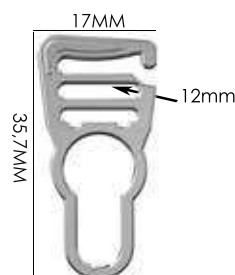
Ref.: AMESP 003 10/13mm Material: zamac Banho: Ouro 24K, Ouro Rosé, Níquel Ouro Velho, Cobre, Latão, Onix, Silver, Prata Velho, Dourado e Light Gold Matte. Espessura: 2,3mm. I Embalagem: 200
