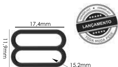
Ref.: APR 025 14mm Espessura: 1.5mm Materiais: POM Embalagem: 1000 unidades
