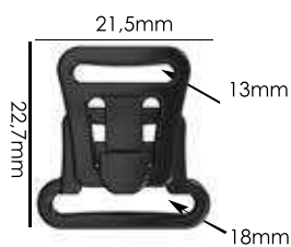
Ref.: APS 001 13 e 18mm espessura: 5mm Materiais: POM e PC Embalagem: 500 unidades
